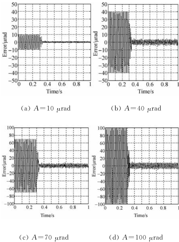
图 3 f = 60 \text{ Hz} 时的实验结果
