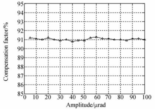
图 4 补偿因子与振幅的关系
